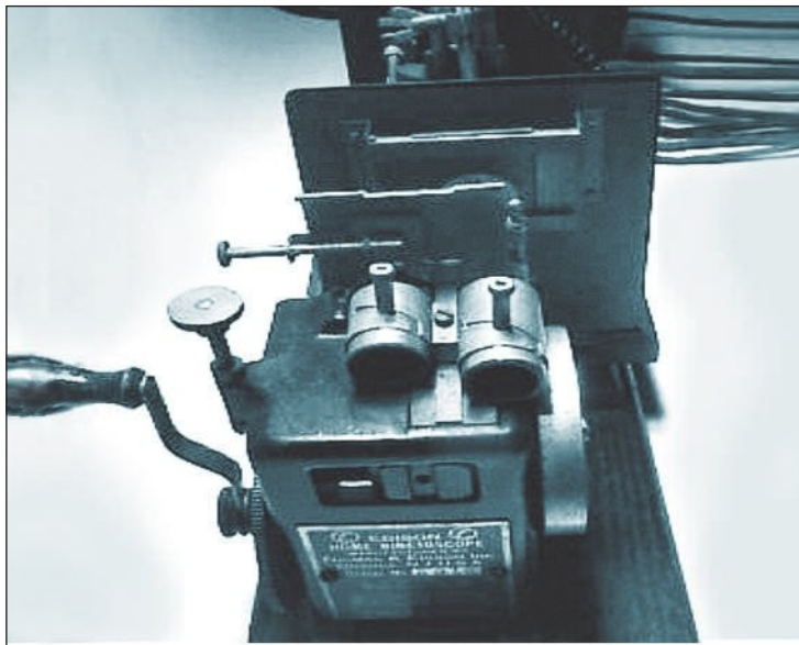
Le kinétoscope (1888) - machine à produire des films par succession rapide de vues individuelles.
