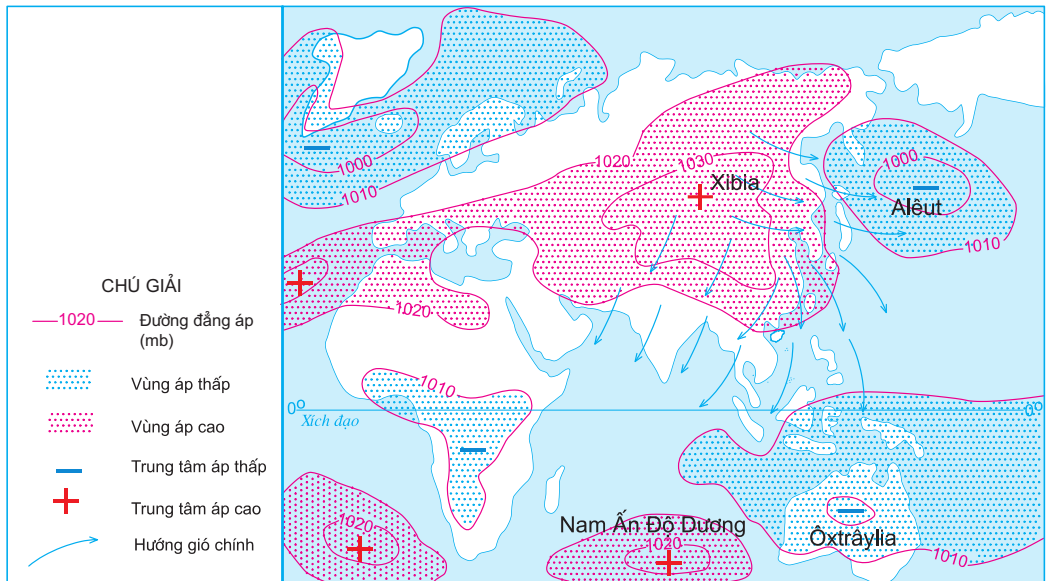
Hình 10.1. Gió mùa đông ở khu vực Đông Nam Á
