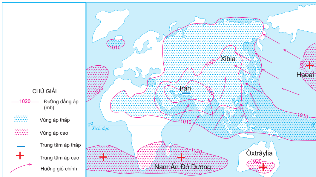
Hình 10.2. Gió mùa mùa hạ ở khu vực Đông Nam Á
