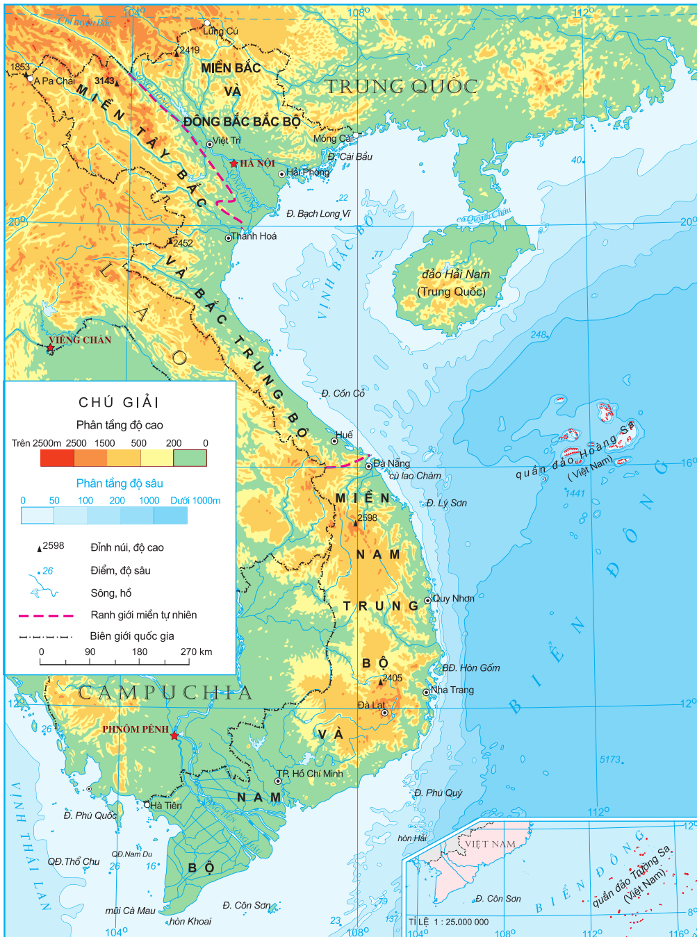
Hình 15. Các miền địa lí tự nhiên
